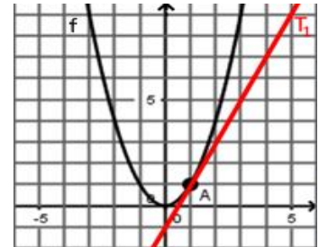
Fig 3 : Une courbe et sa tangente en 1 f'(1) = pente de T_1 = 2
