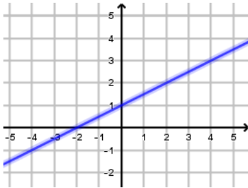
Fig 1 : Droite : y = \frac{1}{2}x + 1 Sa pente est constante égal à 0.5
